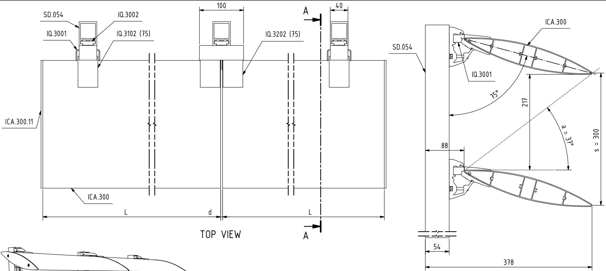
A-A
